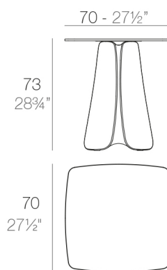
PEZZETTINA Mesa 70x70 PEZZETTINA Dinning Table 27½"x27½"
